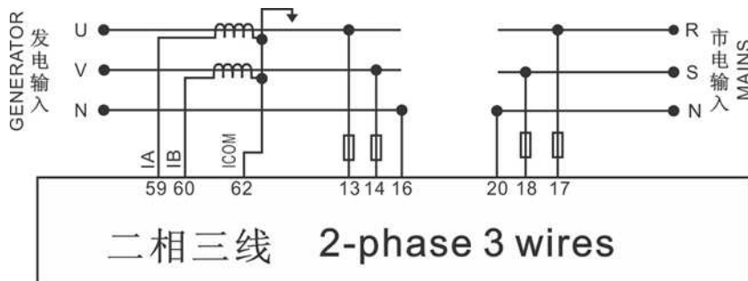
二相三线连接时接线图 (以 LXC9220 为例)
