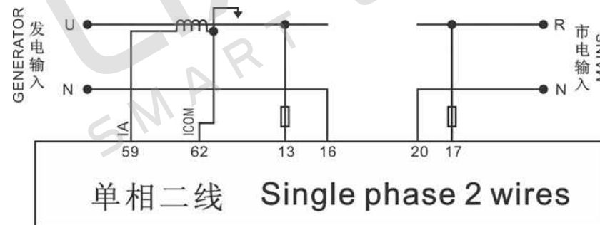
单相二线连接时接线图 (以 LXC9220 为例)
